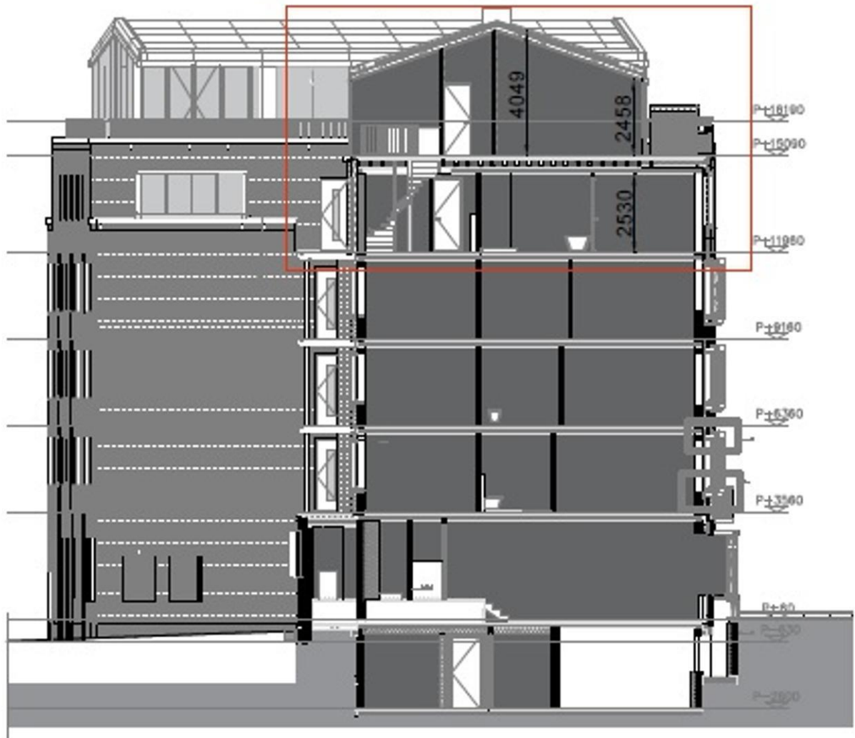
doorsnede A-A'
