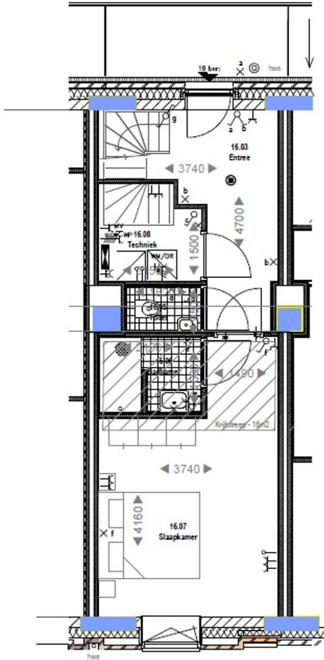
vierde verdieping
